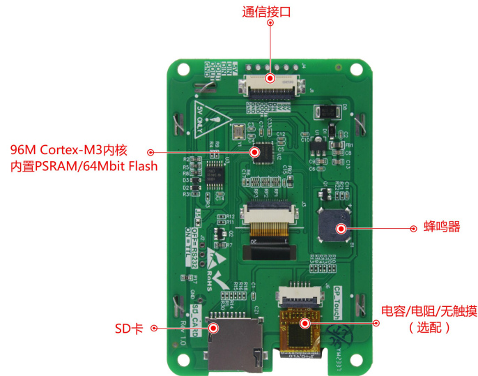
图 1-3 硬件配置图
