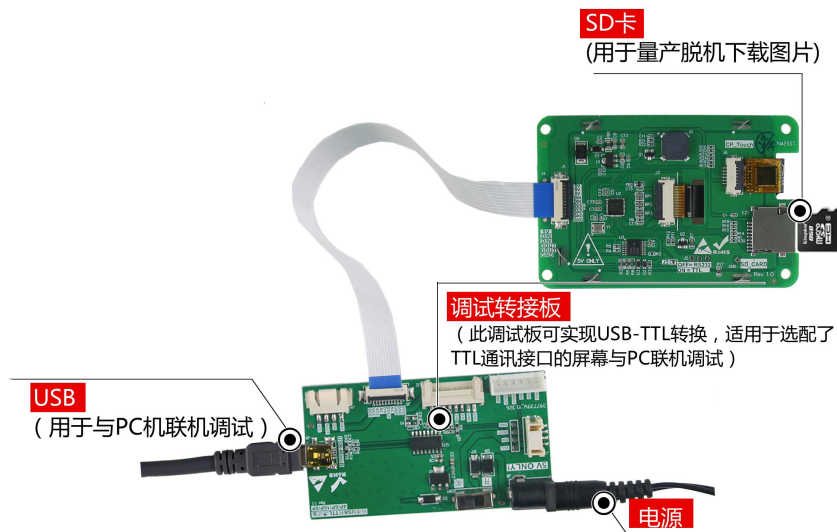
图 1-4 调试工具图
